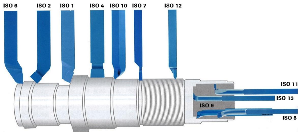
Ilustración 6 Ejemplo de las diferentes operaciones en una sola pieza
