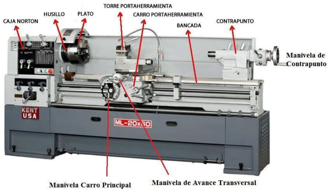
Ilustración 4 Partes del torno
