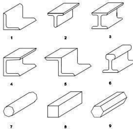
Ilustración 13 Distintos tipos de perfiles
