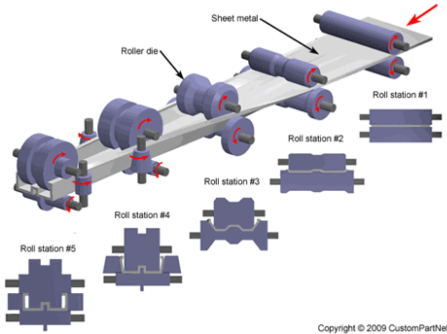
Ilustración 10 Etapas de Producción de perfil
