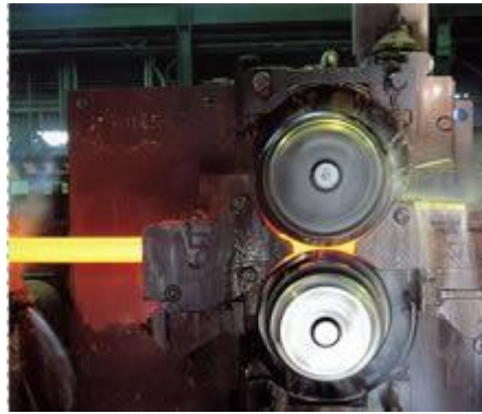
Ilustración 5 Vista del par de rodillos
