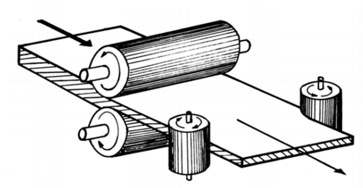
Ilustración 4 Caja de par de rodillos
