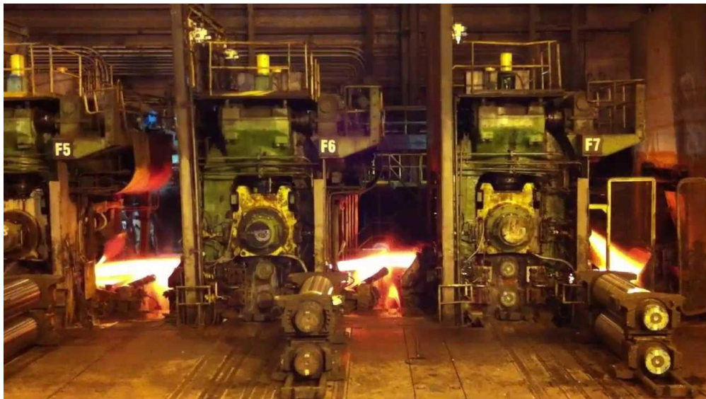
Ilustración 1 Tren de laminación
